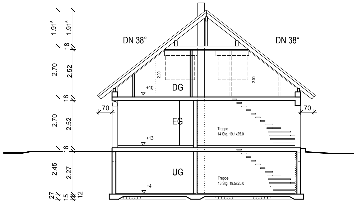
SCHNITT 1-1
