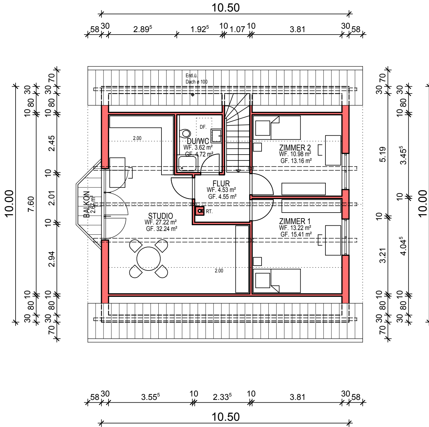
HAUS 142 DACHGESCHOSS-2 M.1:100
