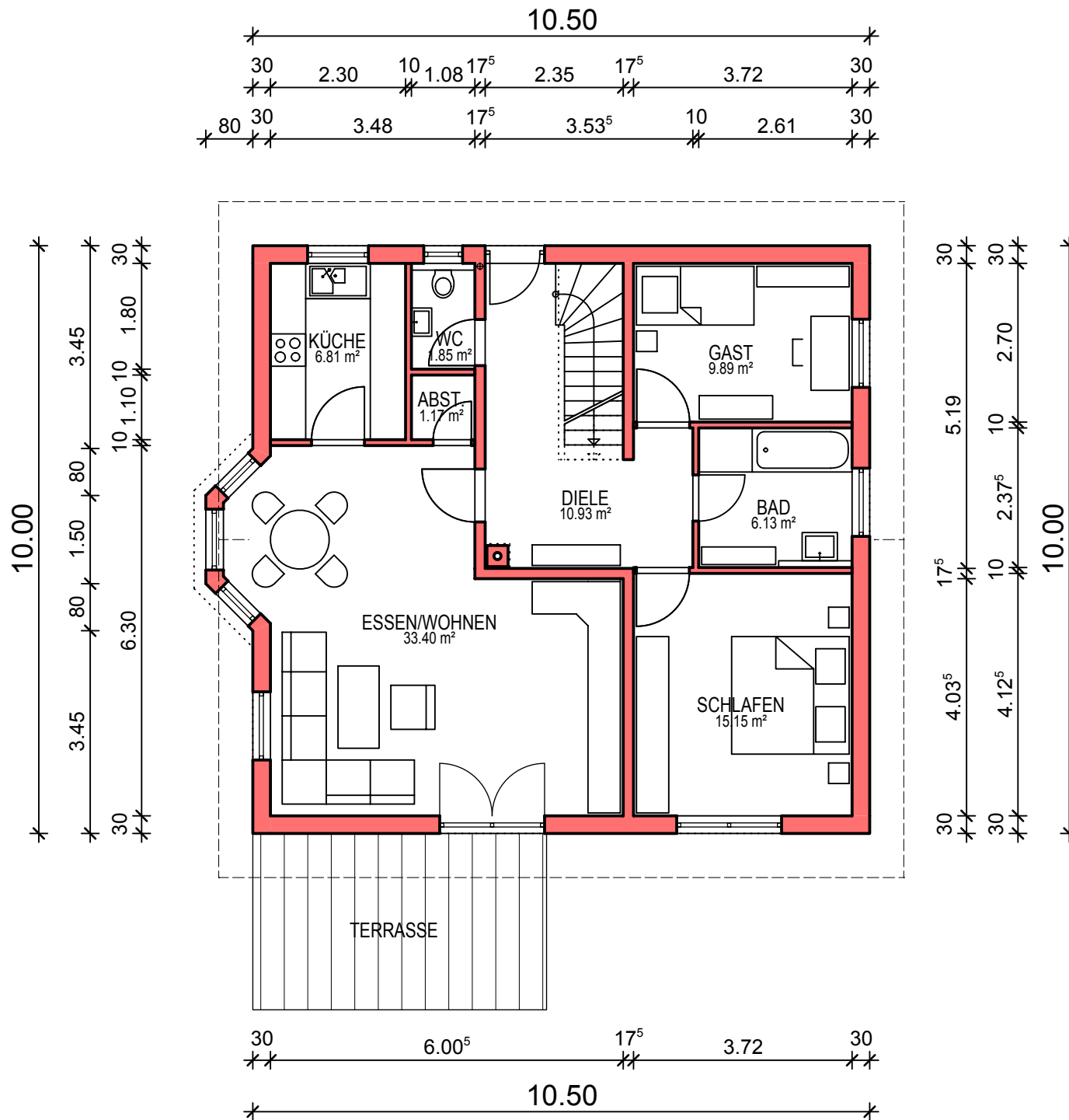
HAUS 142 ERDGESCHOSS M.1:100
