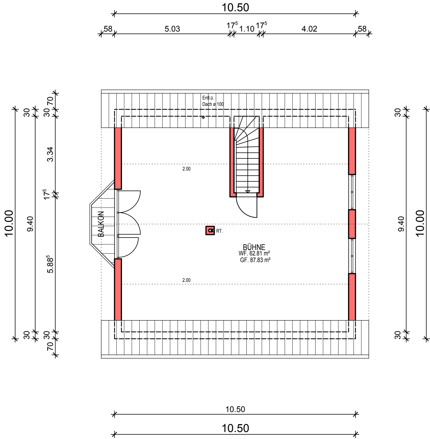
HAUS 142 DACHGESCHOSS-1 M.1:100
